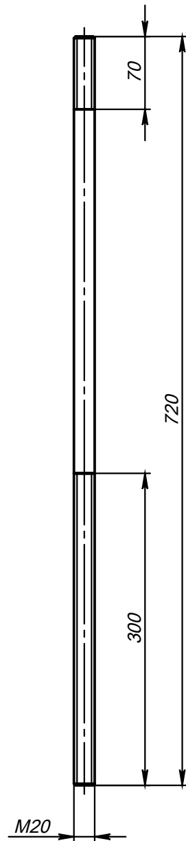
Поз.4 (Шпилька)
